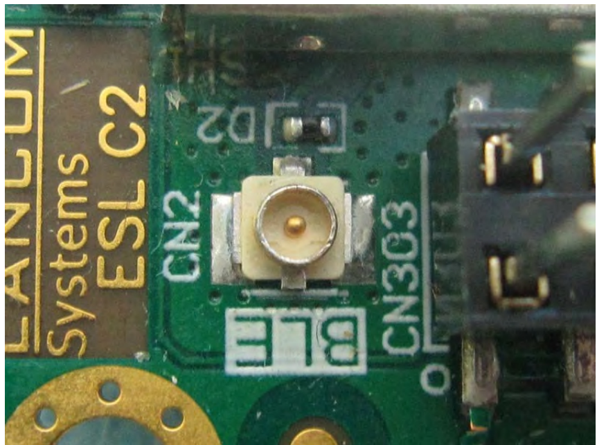
BLE connector
