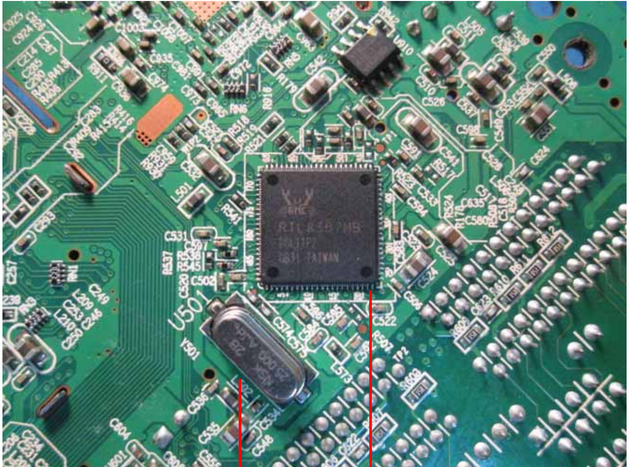
Crystal 25MHz
