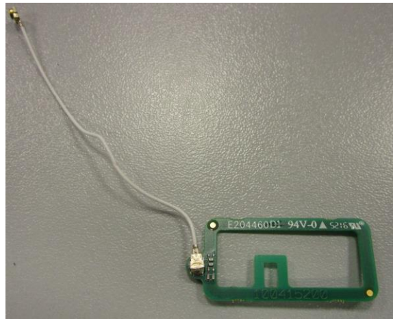
NFC Passive tag
