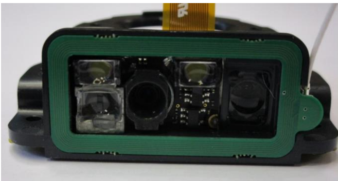
NFC Passive tag
