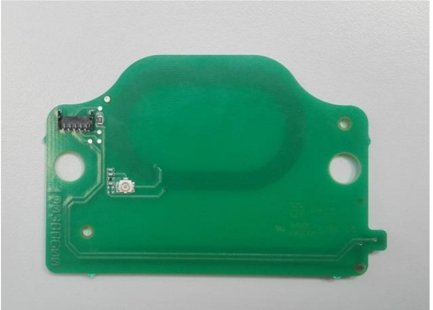
NFC Tx Antenna
