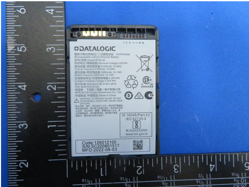
(2) EUT Photo (Battery 1#)
