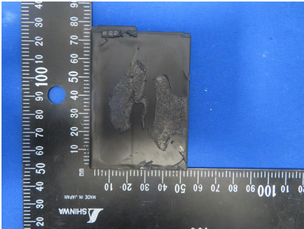
(7) EUT Photo (Battery 2#)
