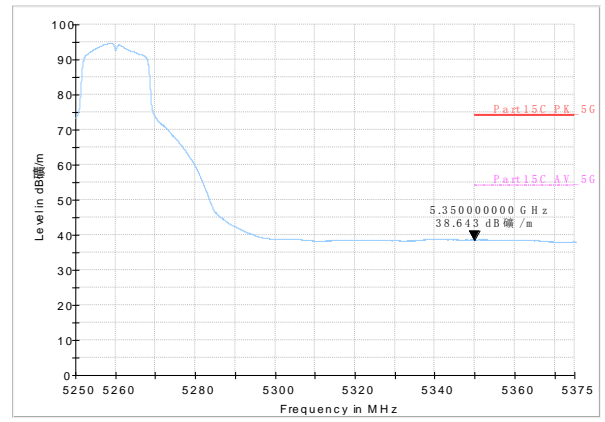
AV detector
