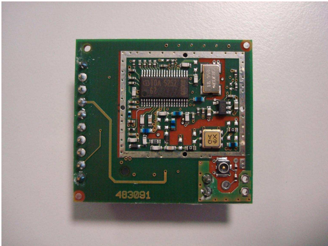
Star Module Plus 910 MHz
