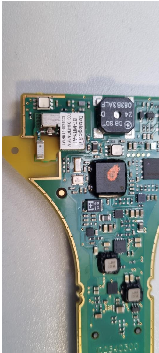
BT module
