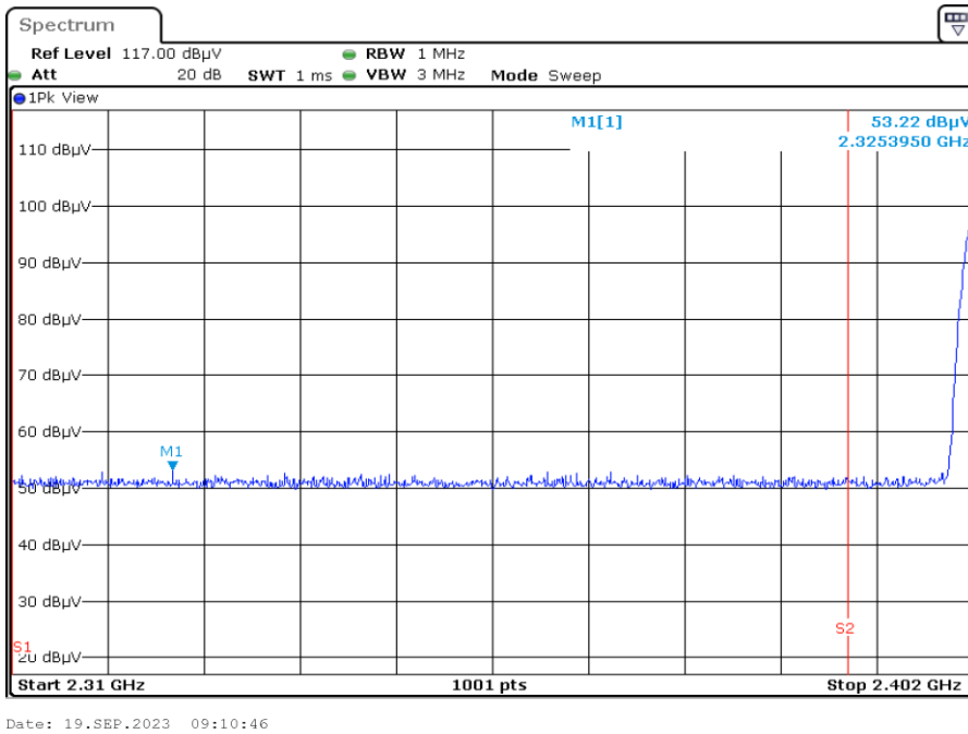
2402.0 F1 RestrictedBand Vertical PEAK
