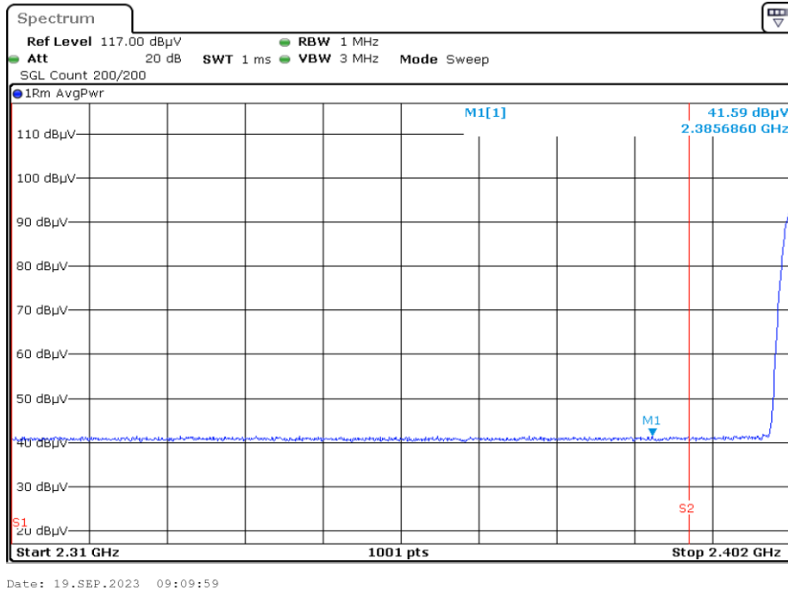
2402.0 F1 RestrictedBand Vertical AVG
