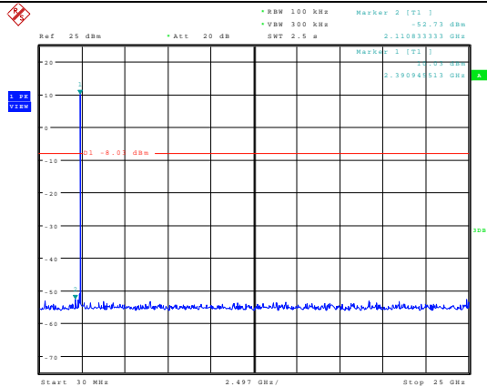
30MHz-25GHz
