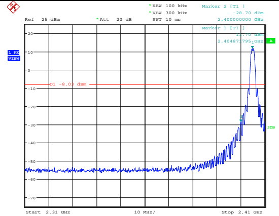
Lower Edge
