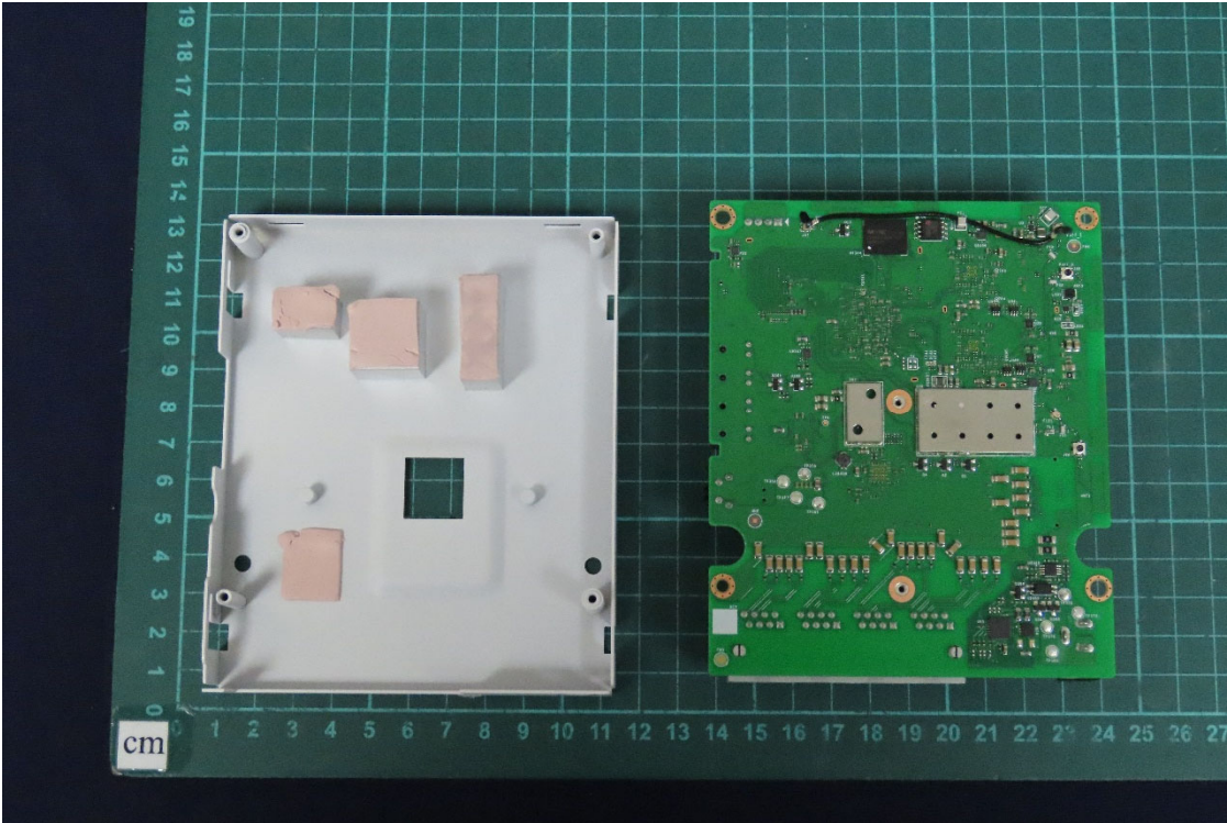
(3) EUT Photo
