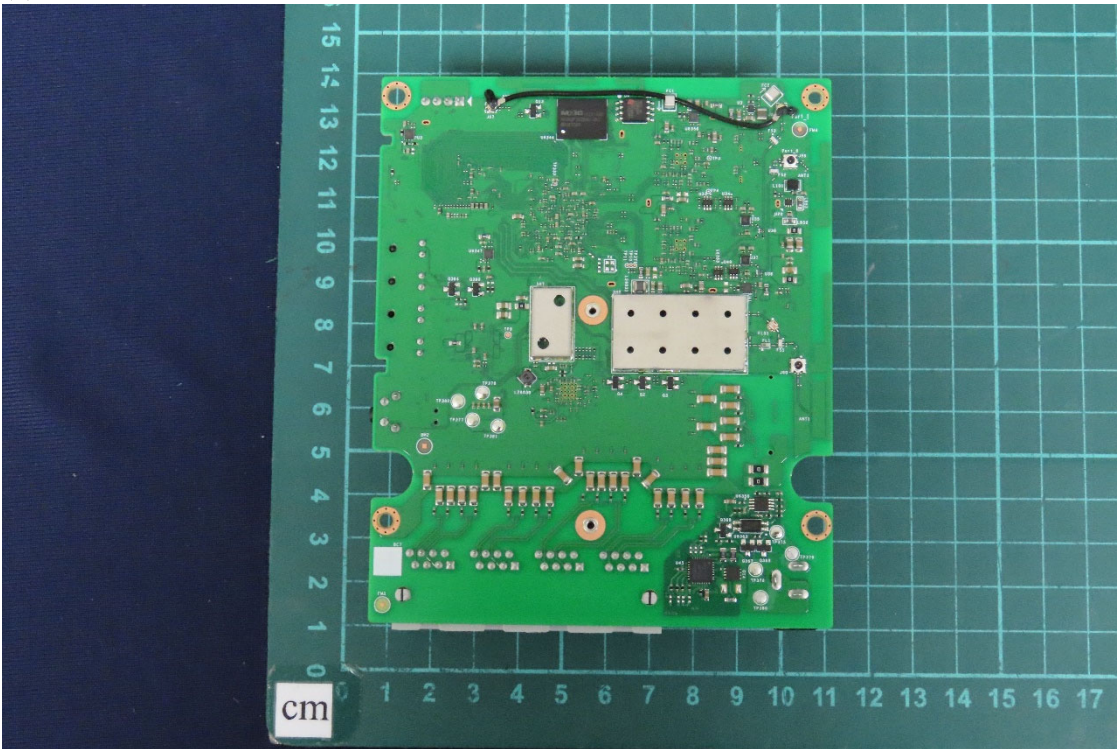
(4) EUT Photo
