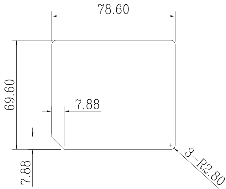
刀模尺寸圖
