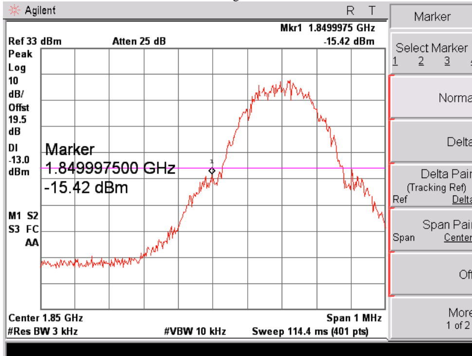
Band edge – Lower
