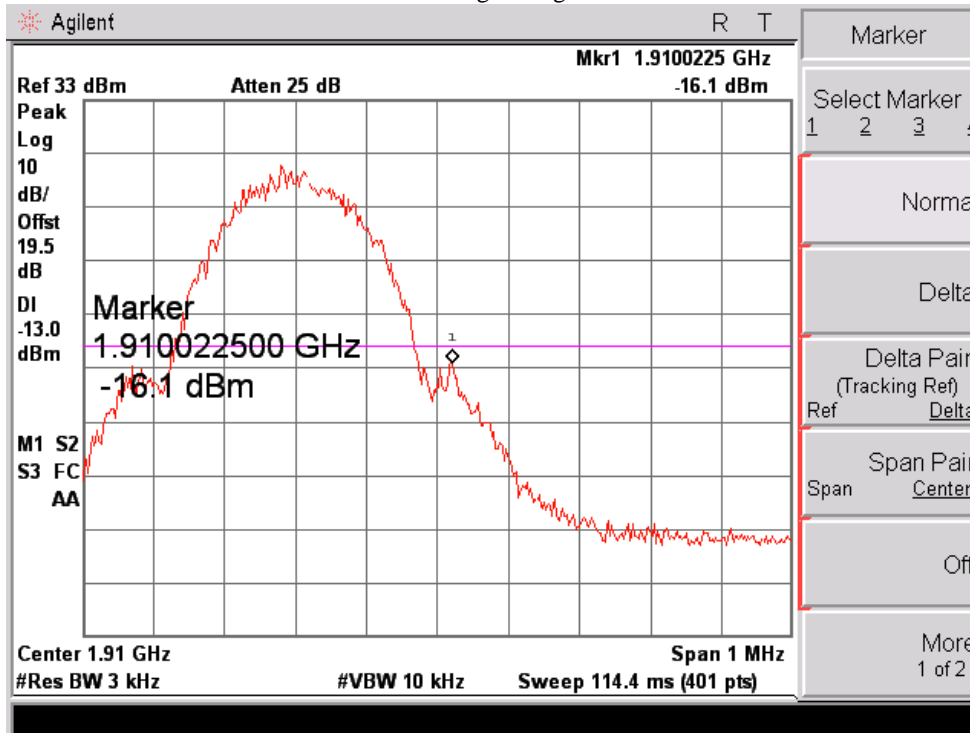
Band edge – Higher
