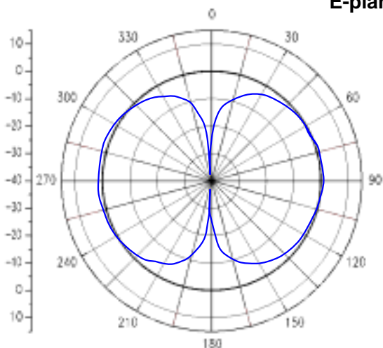
E-plane
