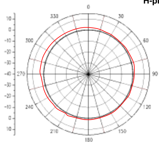
H-plane
