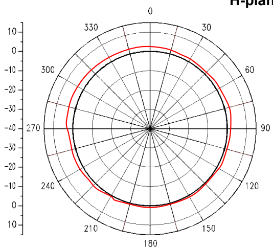
H-plane
