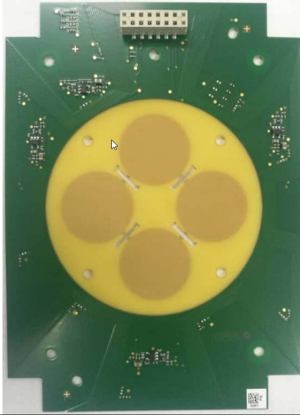
Sensor PCBA, top
