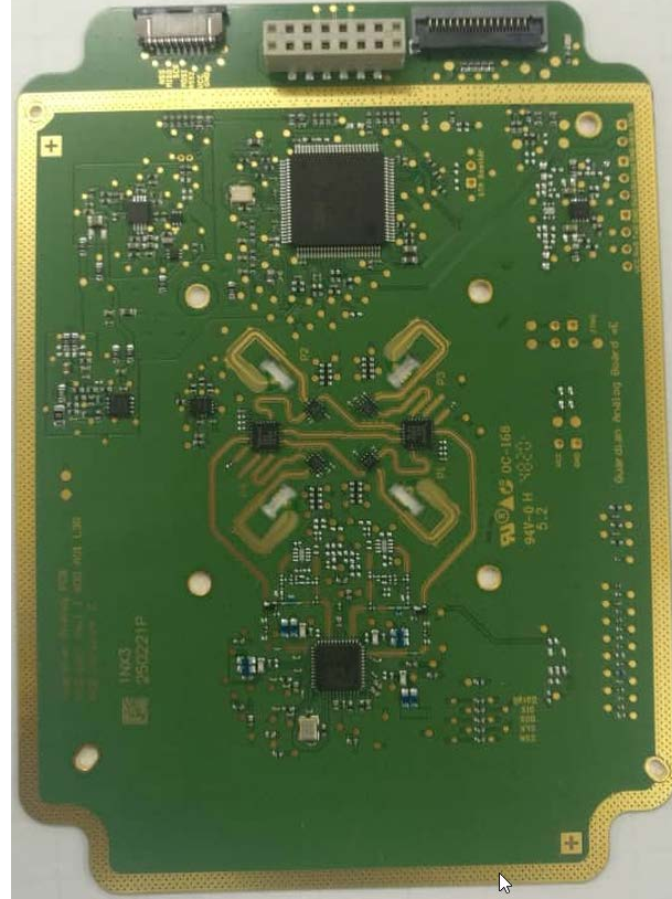
Analog PCBA, top
