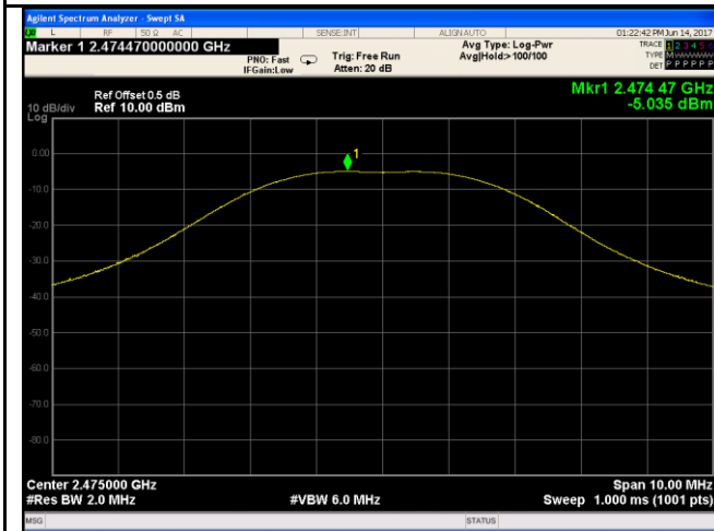
AV Output power - High CH 2475
