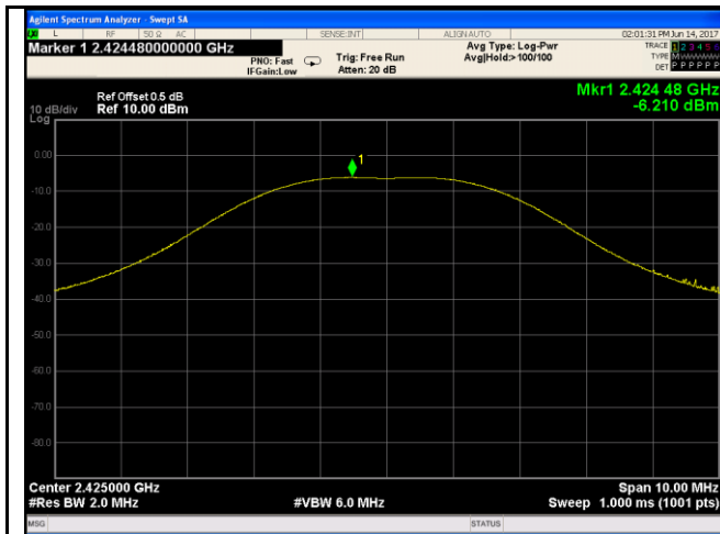
AV Output power - Low CH 2425
