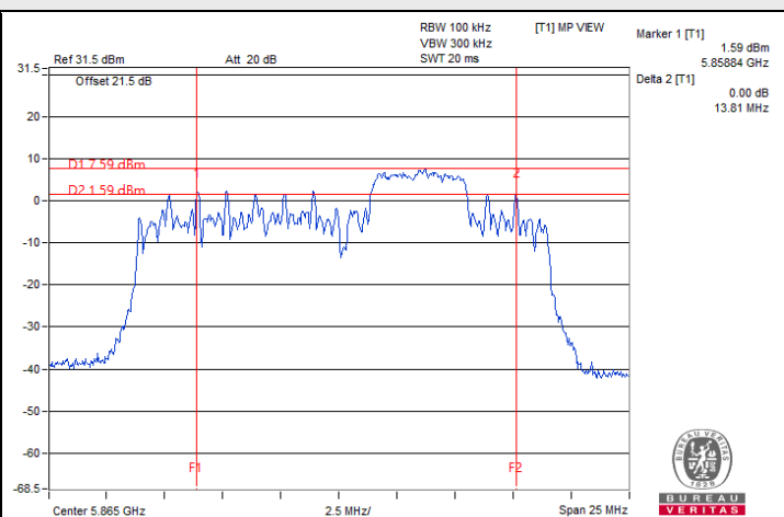
802.11ax (HE) 52-tone RU : CH 173
