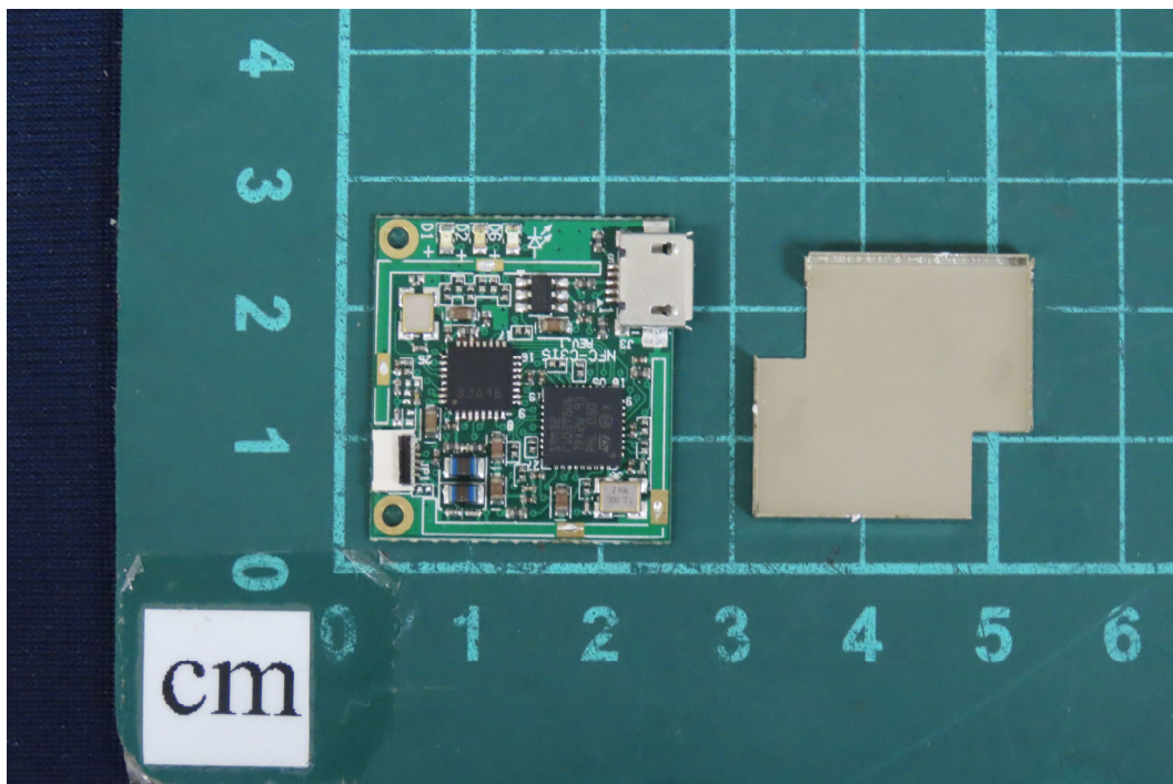
(52) EUT Photo
