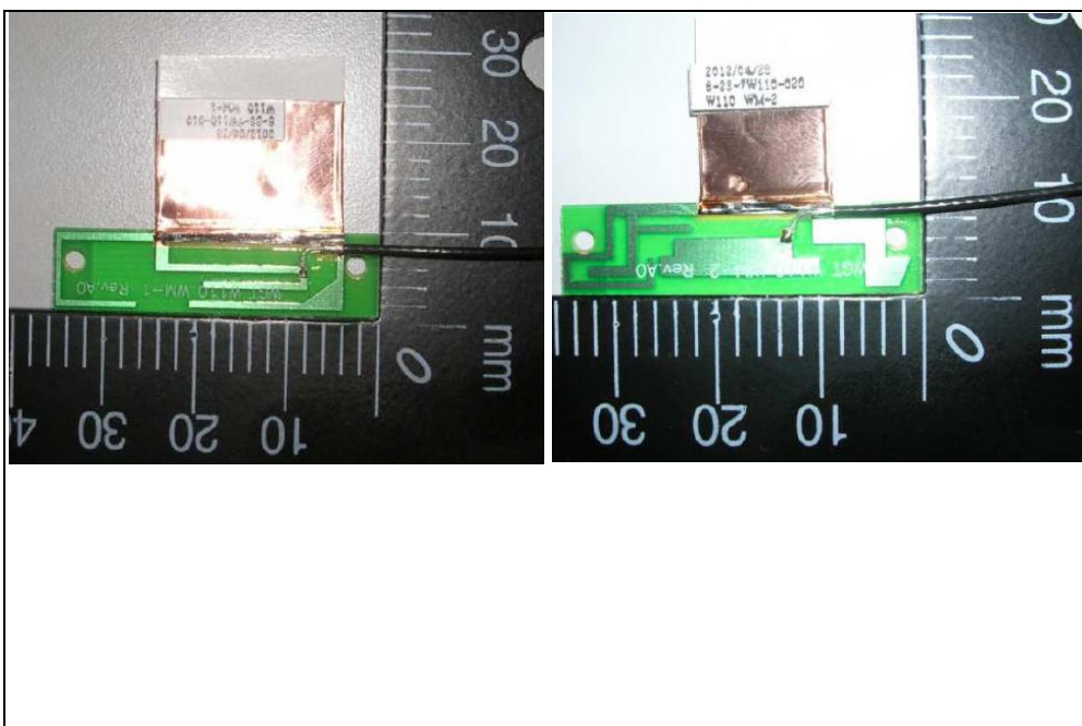
Antenna 10: Brand: WGT / Model: SK110WMPB01+A (Tx1) & SK110WMPB02+A (Tx2)
