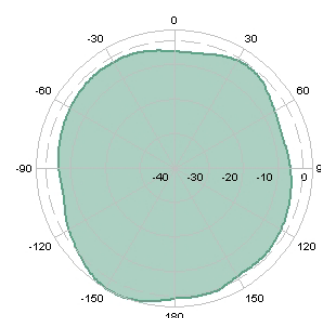
Horizontal 5600MHz
