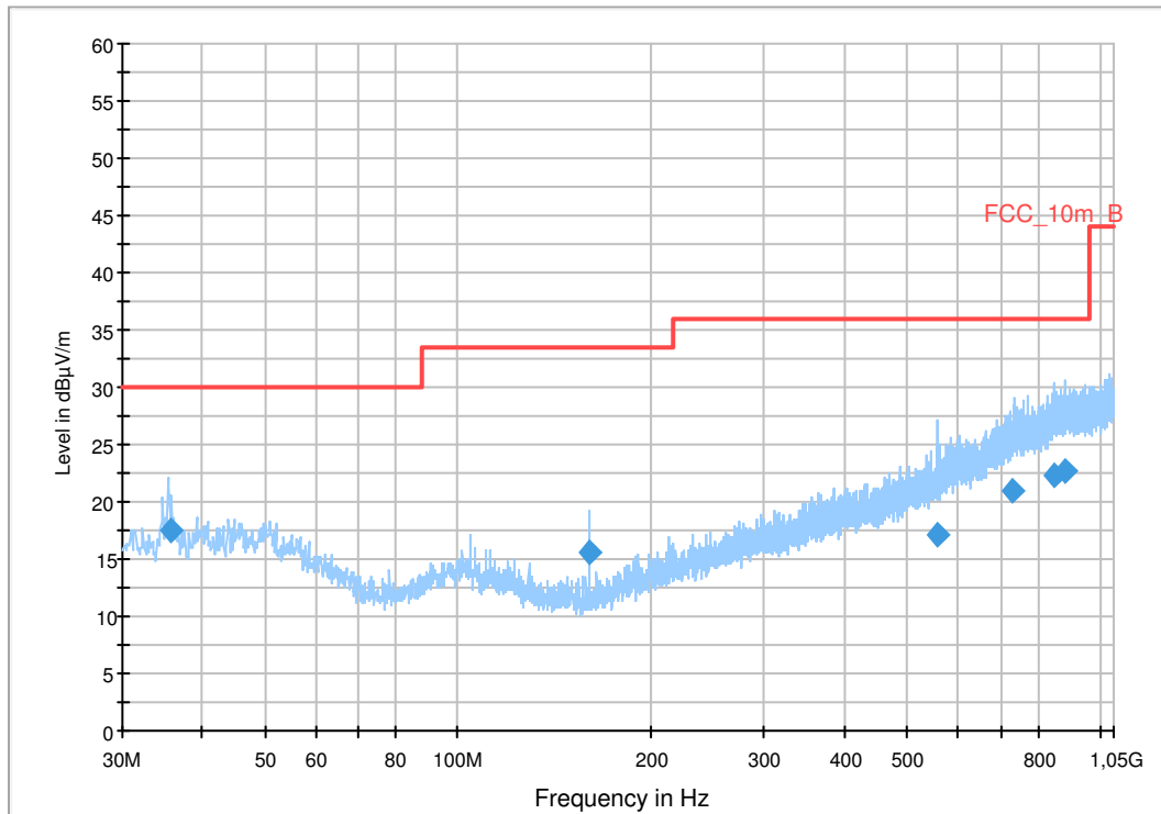
FCC_10m(B)
