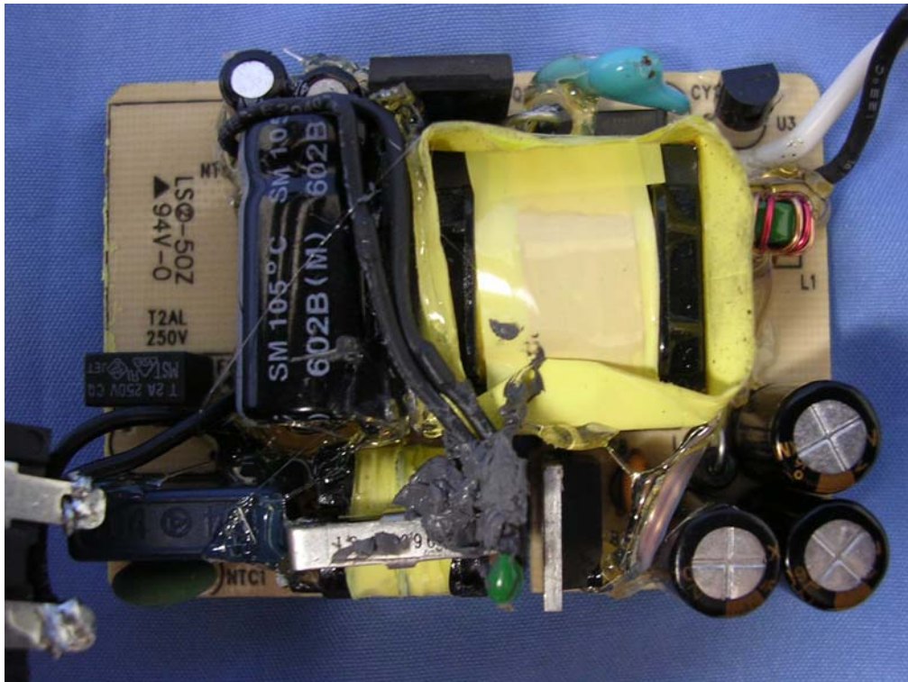
(52) EUT Photo
