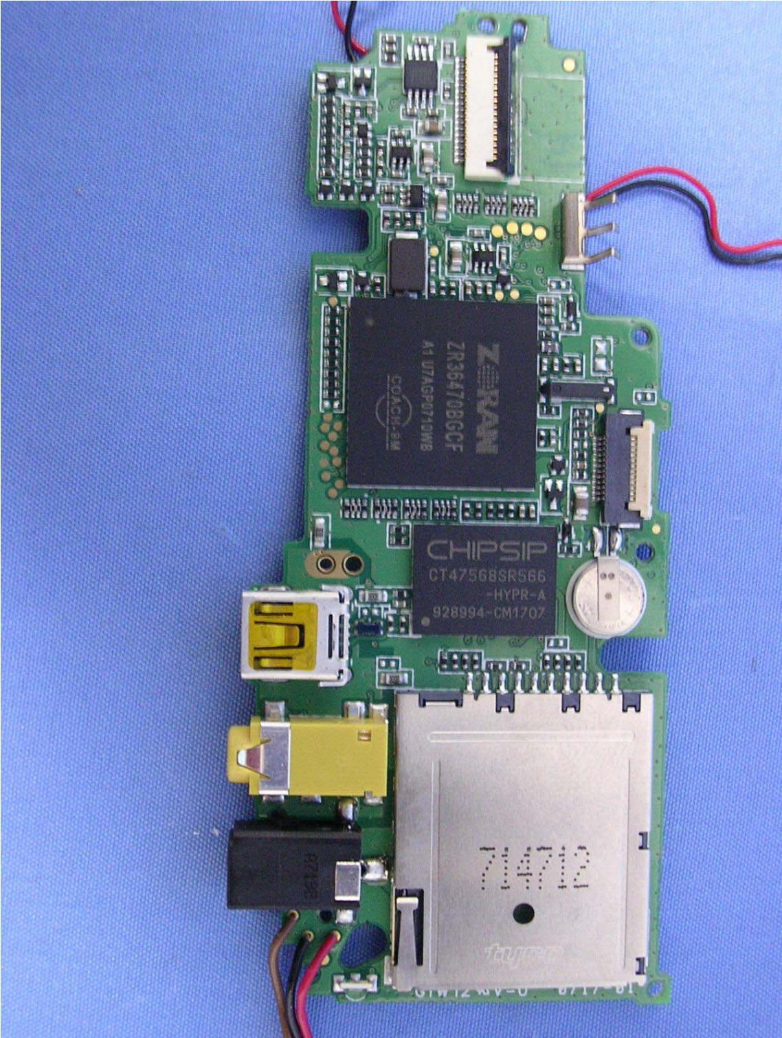
(37) EUT Photo
