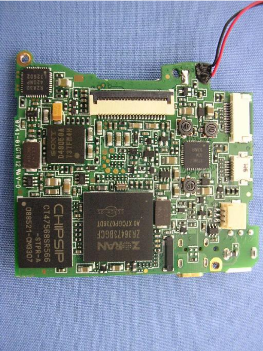
(40) EUT Photo
