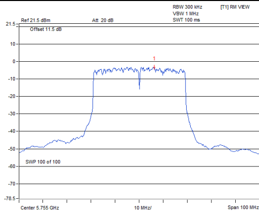
802.11ax (HE40)
