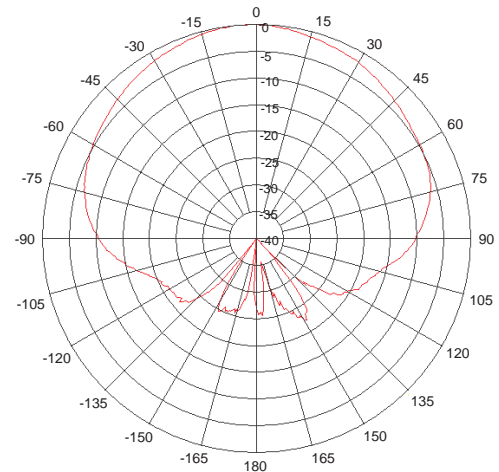
H-Plane Pattern
