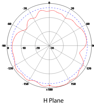
Port 3: 2450MHz
