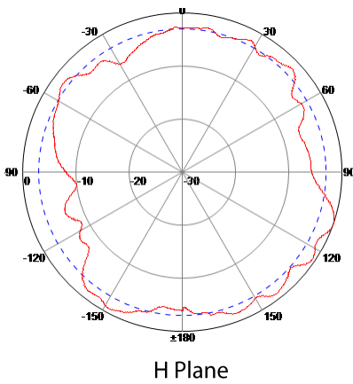
Port 3: 5500MHz
