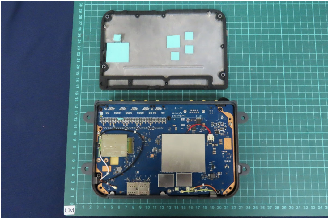
(56) EUT Photo
