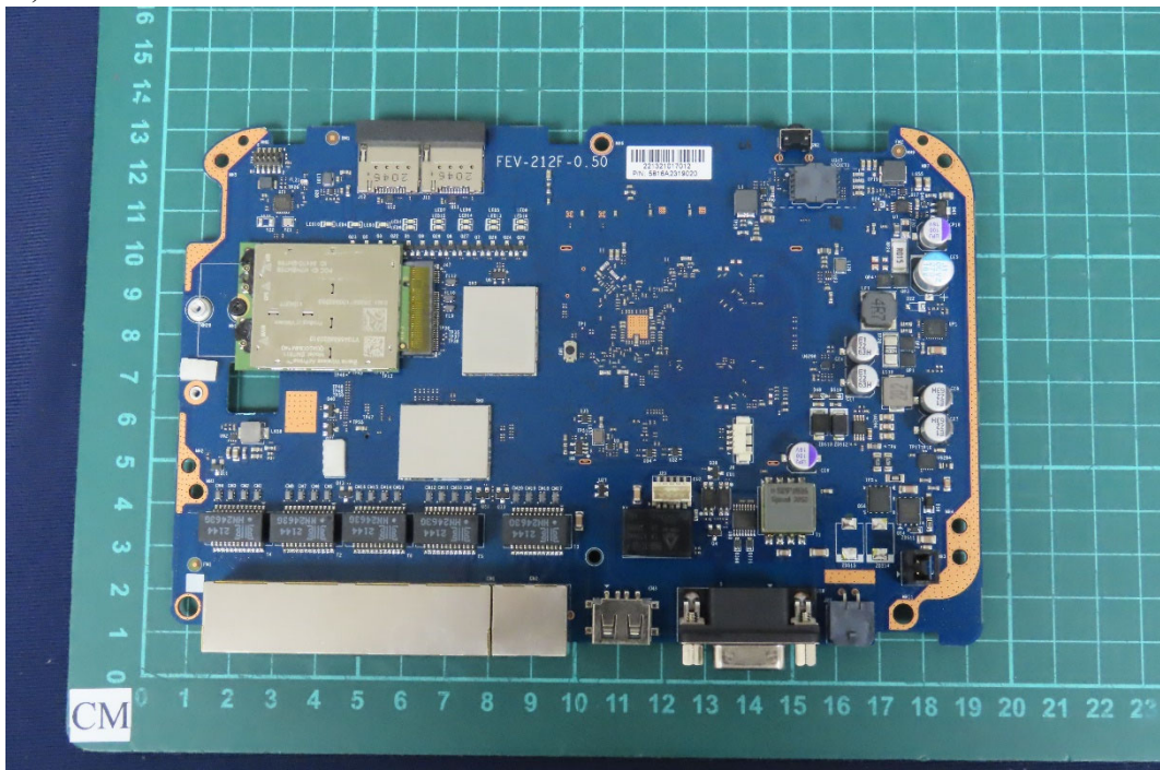
(66) EUT Photo
