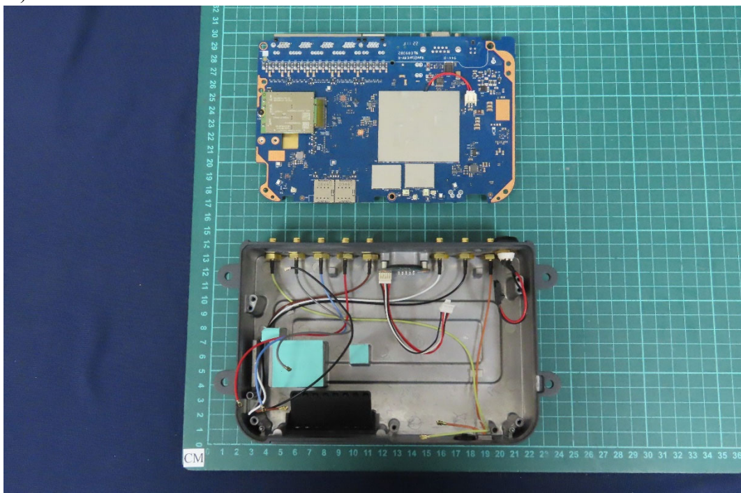
(58) EUT Photo
