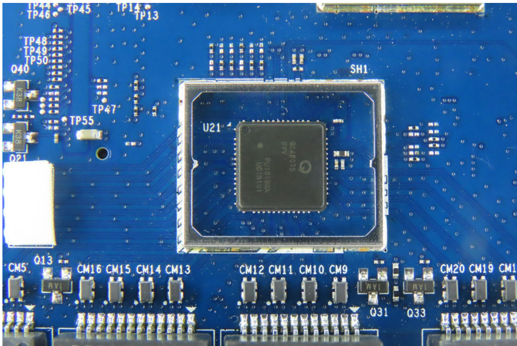
(72) EUT Photo
