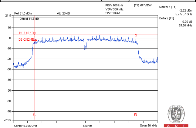
802.11ac (VHT40)
