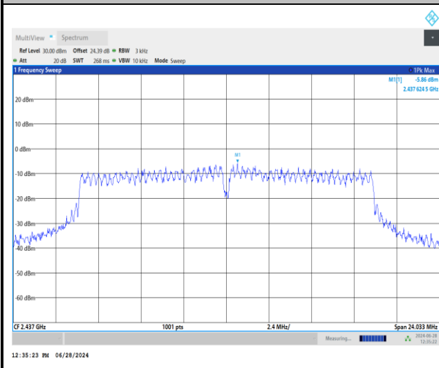
MIMO Ant 1
