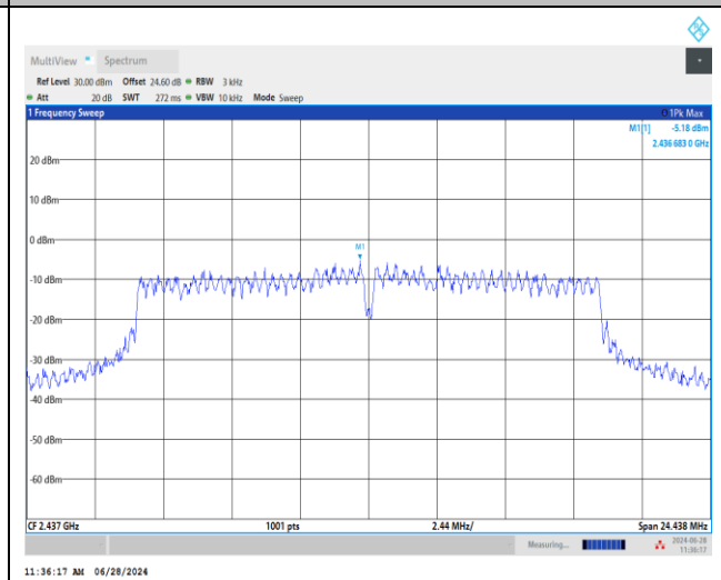
MIMO Ant 2
