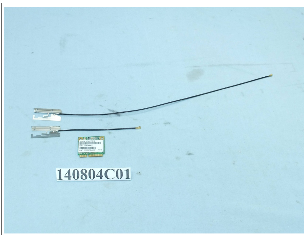
PIFA Antenna Set 1 antenna
