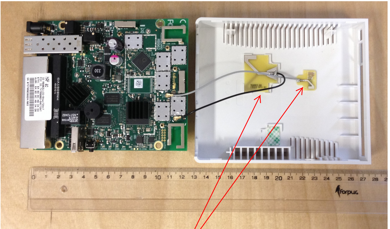
Antennas
