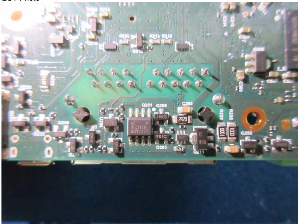
(36) EUT Photo
