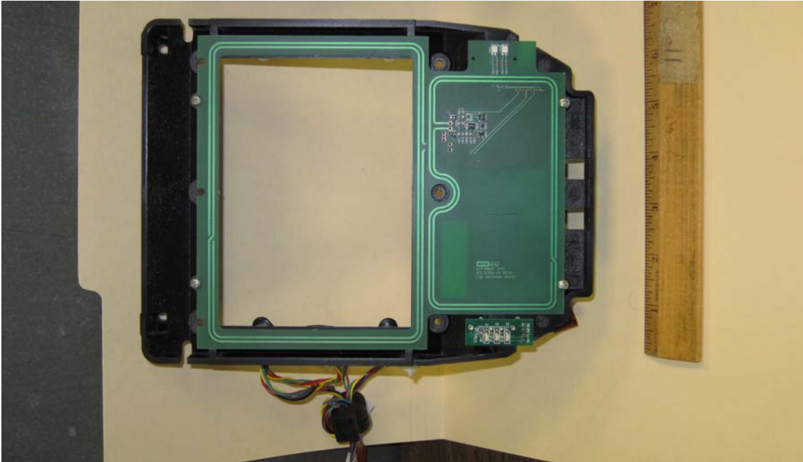
Antenna module
