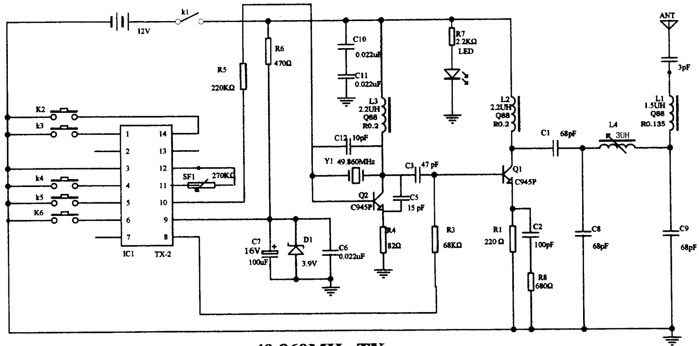
49.860MHz TX
