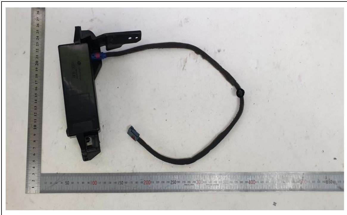
<Pad_Antenna>
