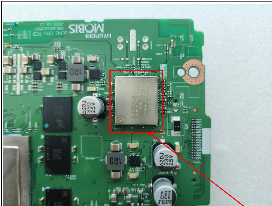
BT/WIFI Module
