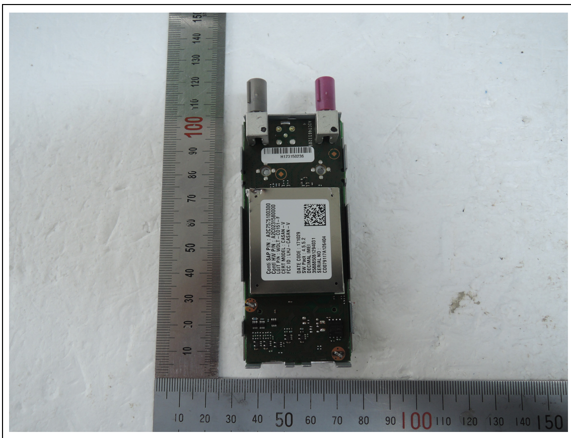
<LTE Module>
