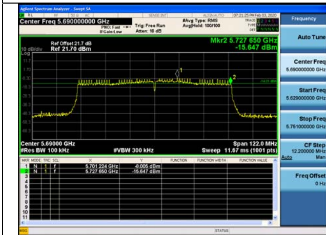
802.11ac_VHT80 CH.138
