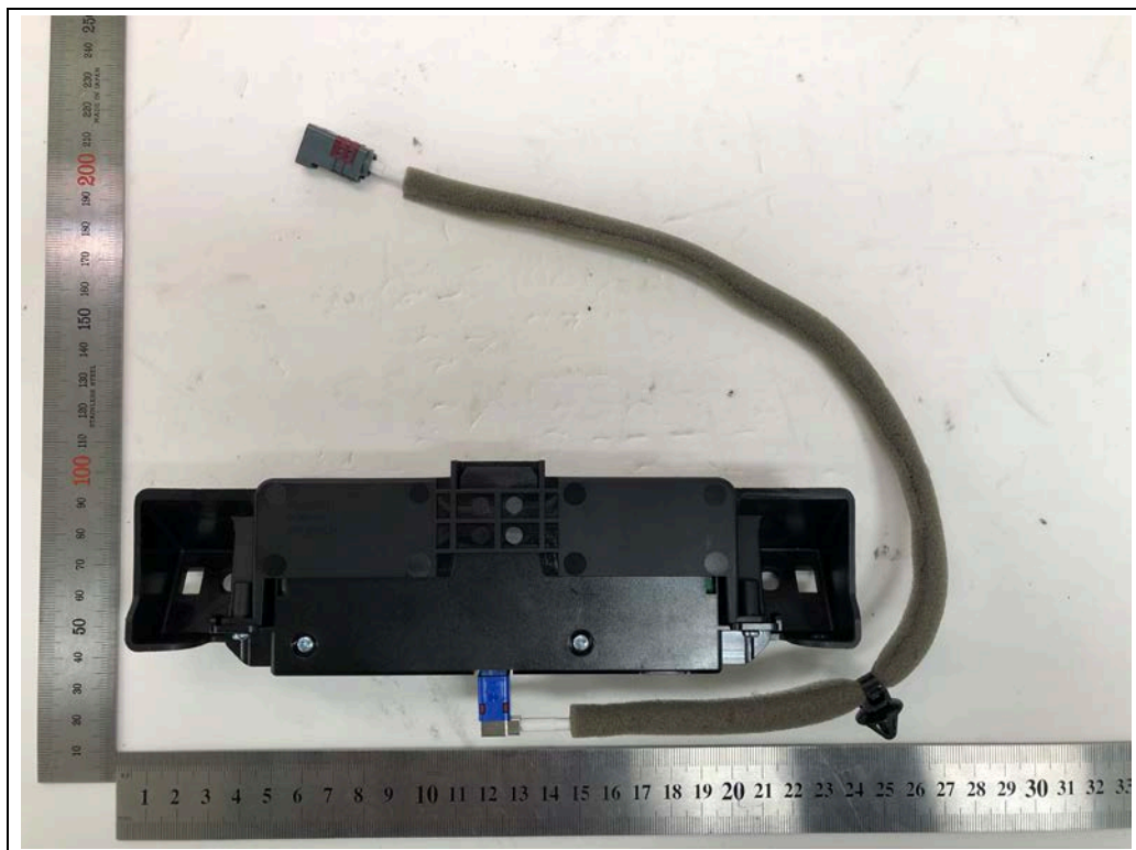
<Antenna Pad_2>
