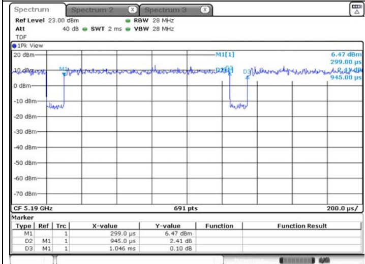
802.11n_HT40
