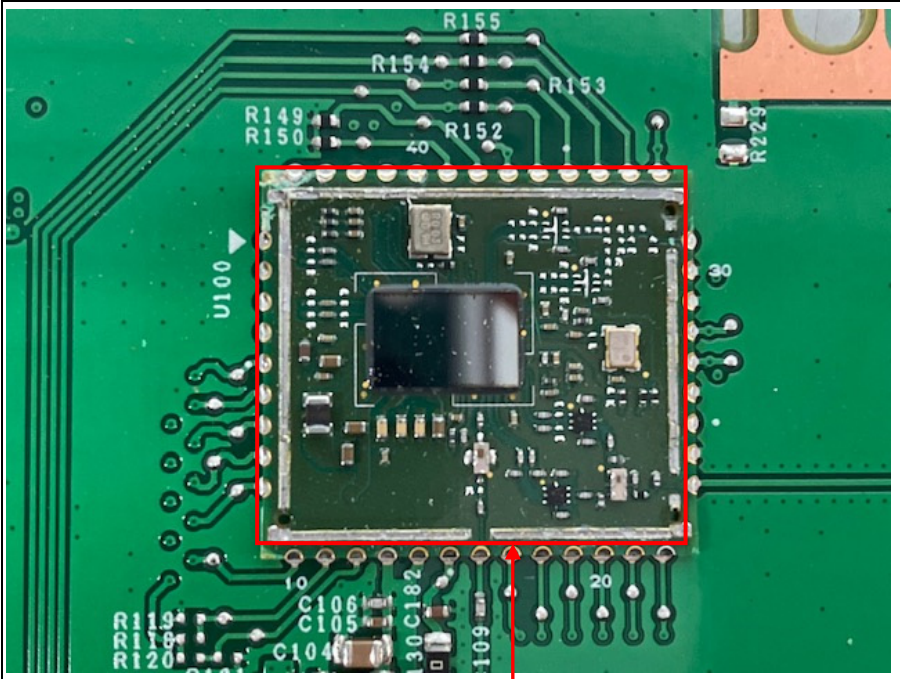
BT/WIFI Module
