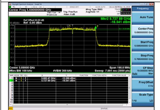
802.11ac_VHT80 CH.138
