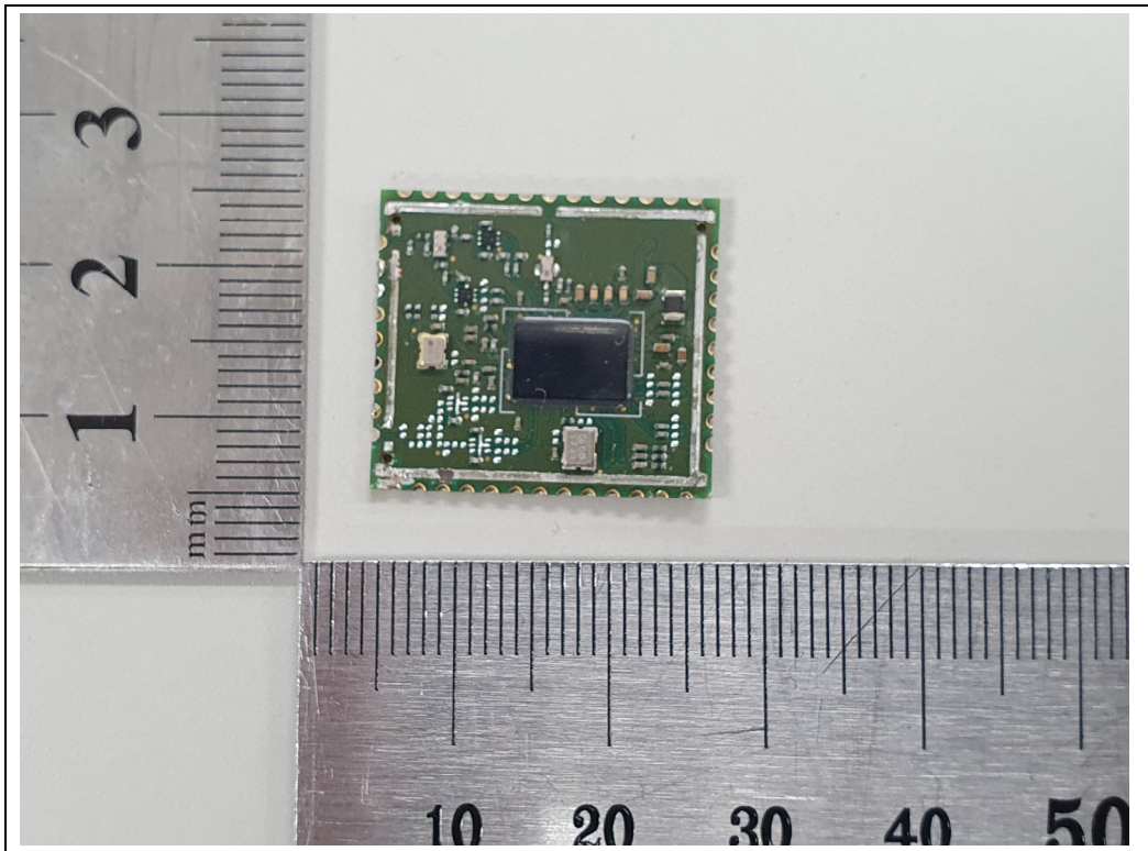
< SUBPCB Module >
