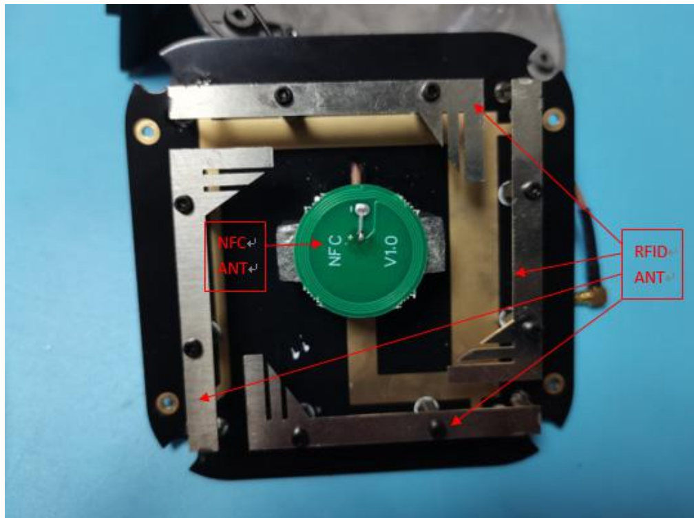
Antenna- RFID&NFC
