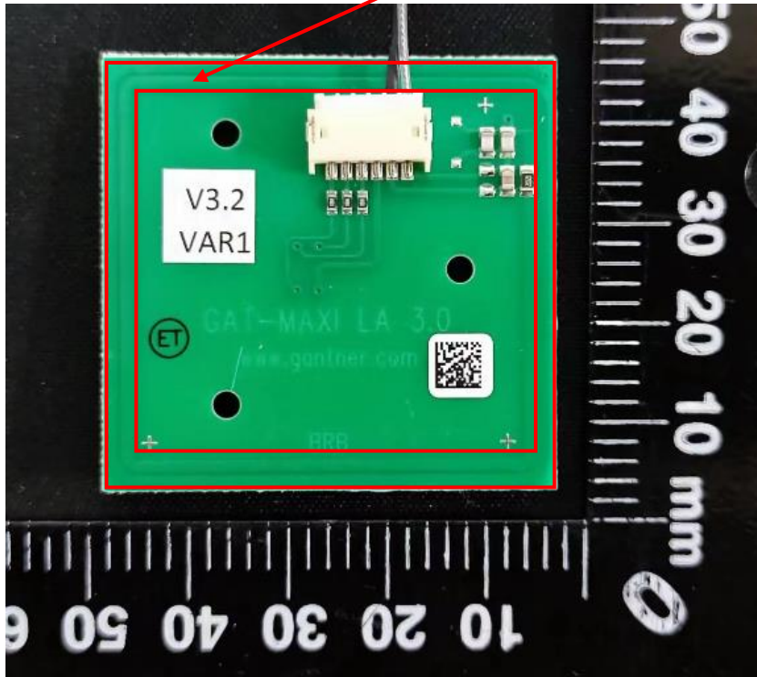
RFID antenna
