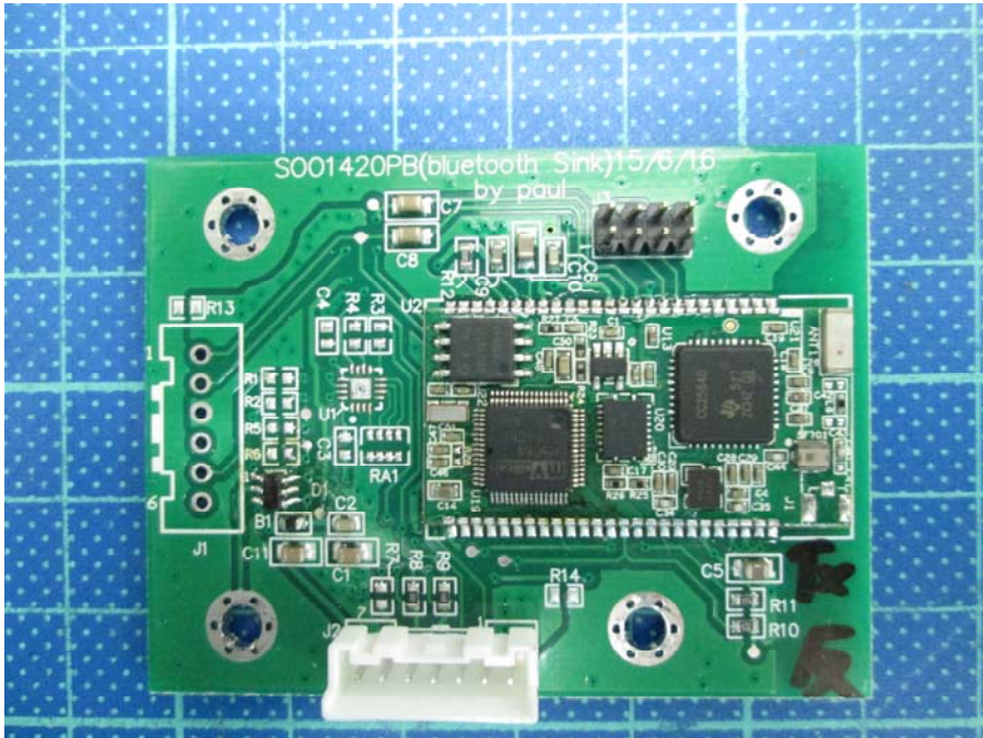
Bluetooth module
