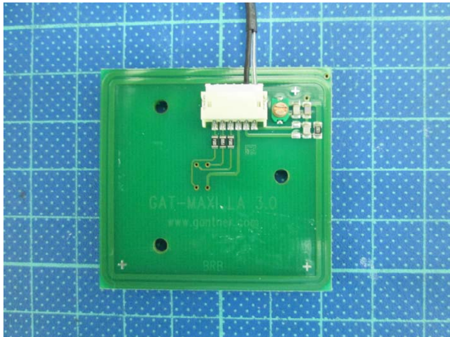
NFC antenna
